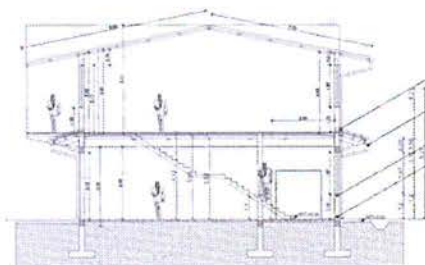
Fig. 6: Corte Esquemático de Bloque Plan Común de 2 niveles. Fuente: Elaboración propia
