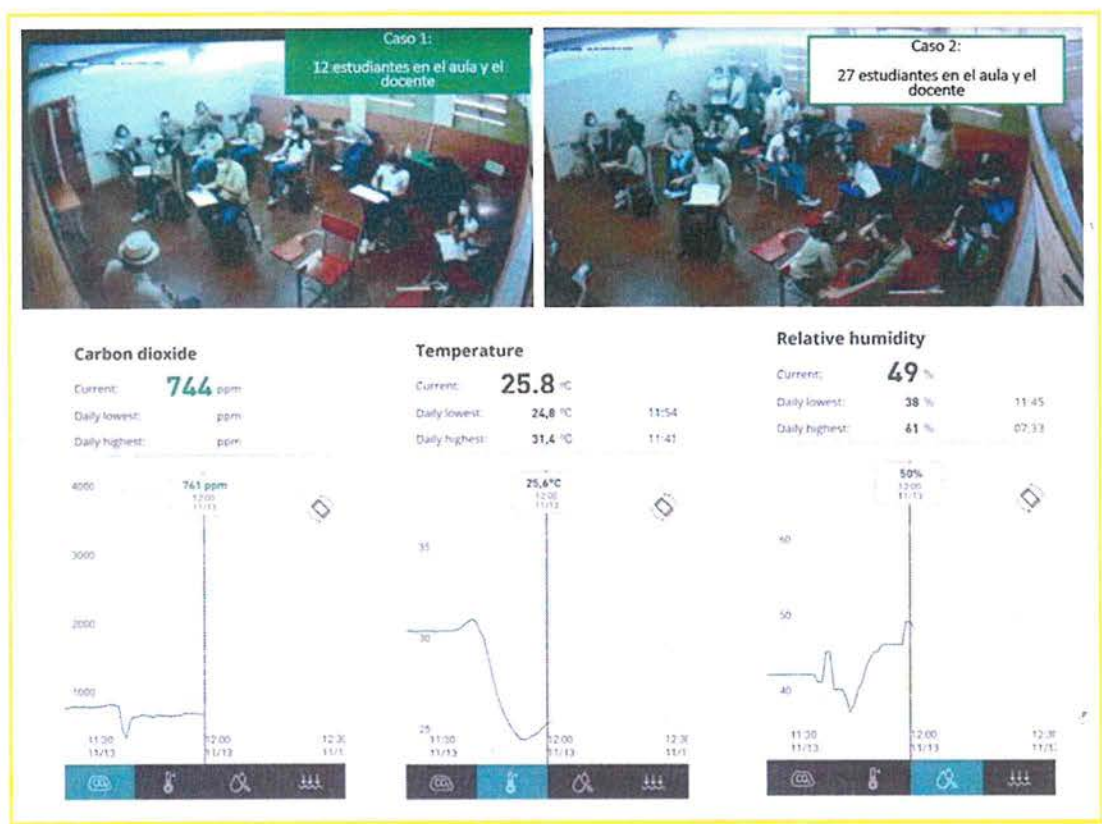
Fig. 4: Estudio 1: Mediciones en Aula 5 CC de 1 nivel. Fuente: Elaboración propia
