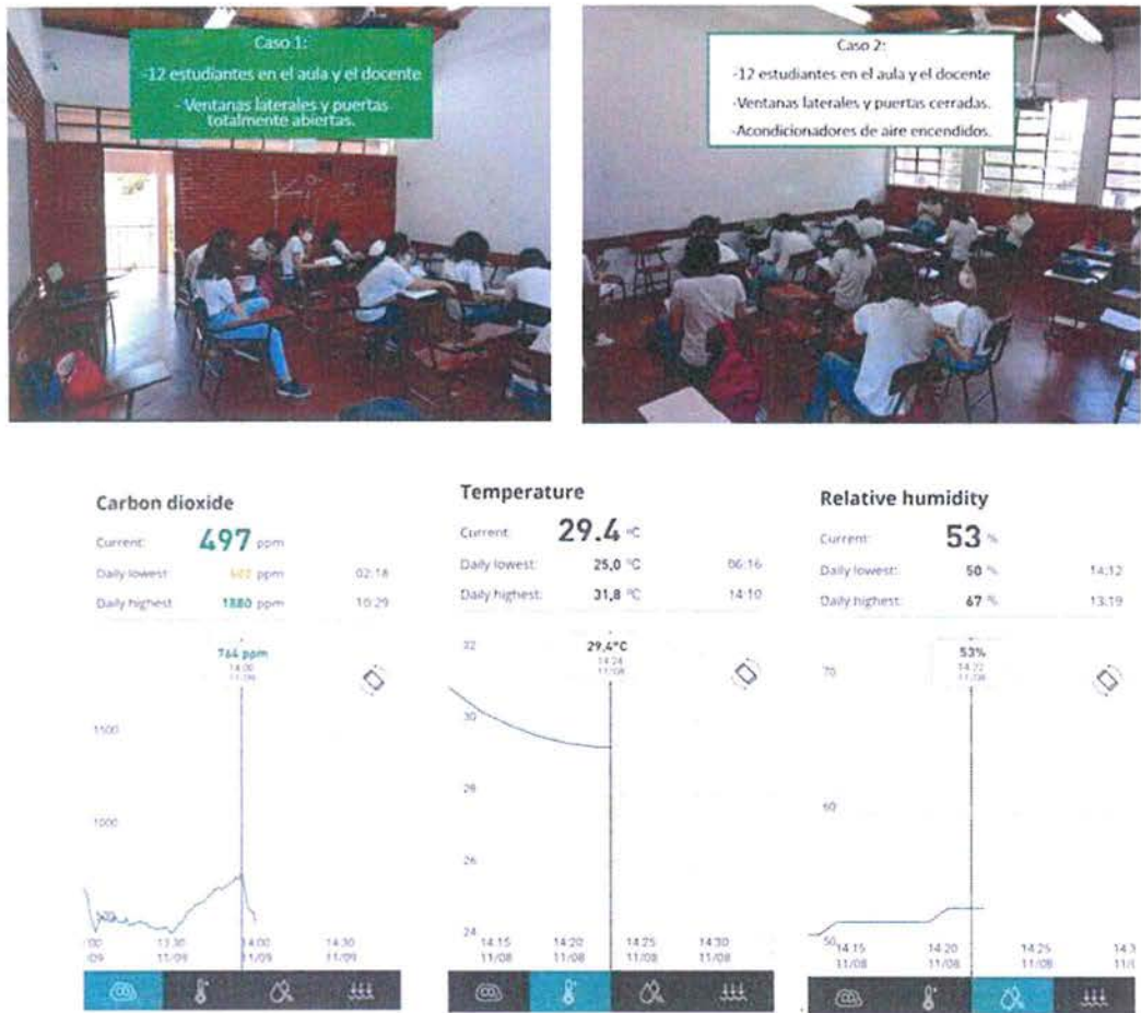
Fig. 5: Estudio 2. Mediciones en Aula 10 Bloque Plan Común de 2 niveles. Fuente: Elaboración propia
